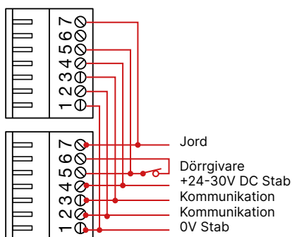
Kopplingsschema för dörlägesgivare
